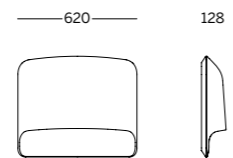
MODULE 2 - Backrest
